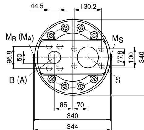
Teilansicht Y
