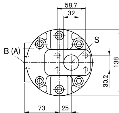
Ansicht Y
